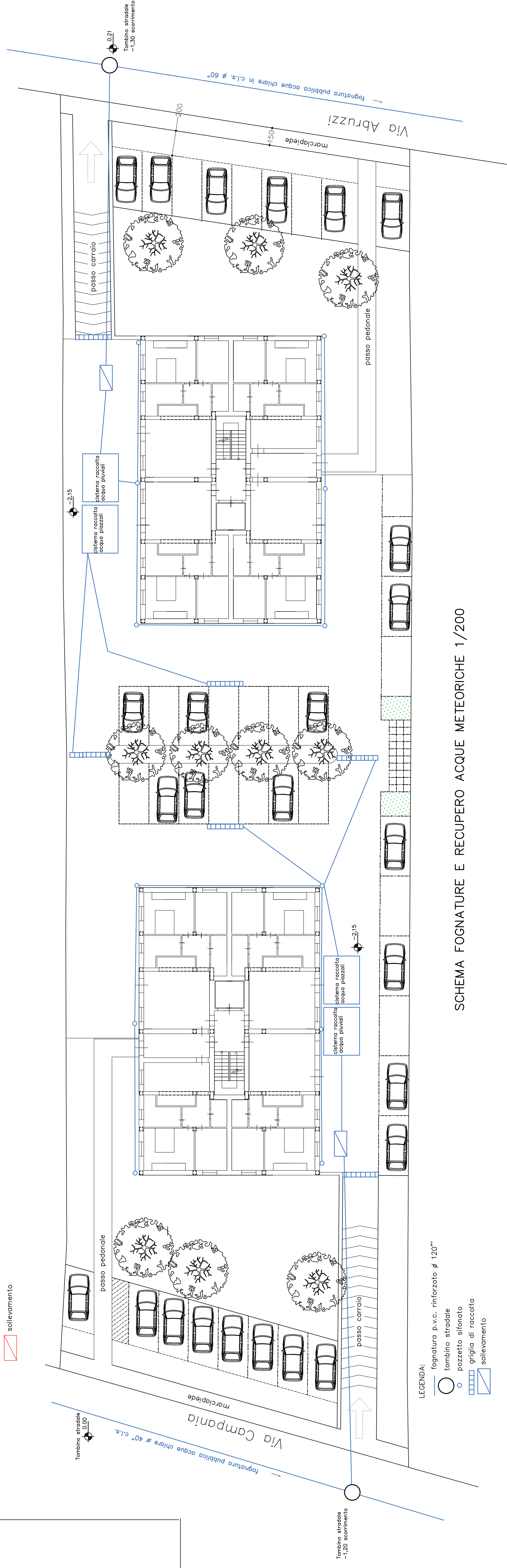
SCHEMA FOGNATURE ACQUE NERE 1/200
