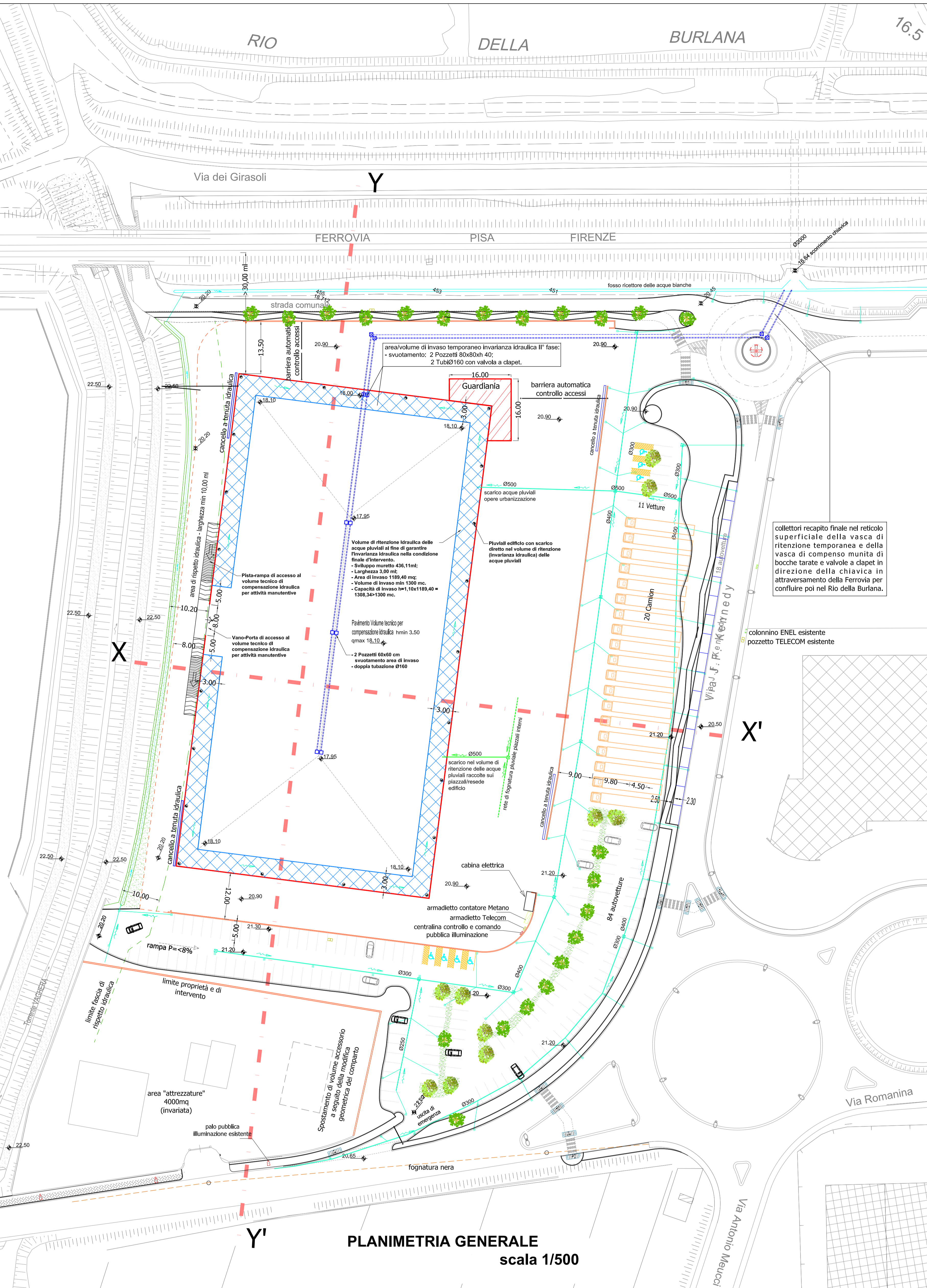
Verifica Invarianza Idraulica - II° Fase: Opere di urbanizzazione realizzate con macrolotto edificato
