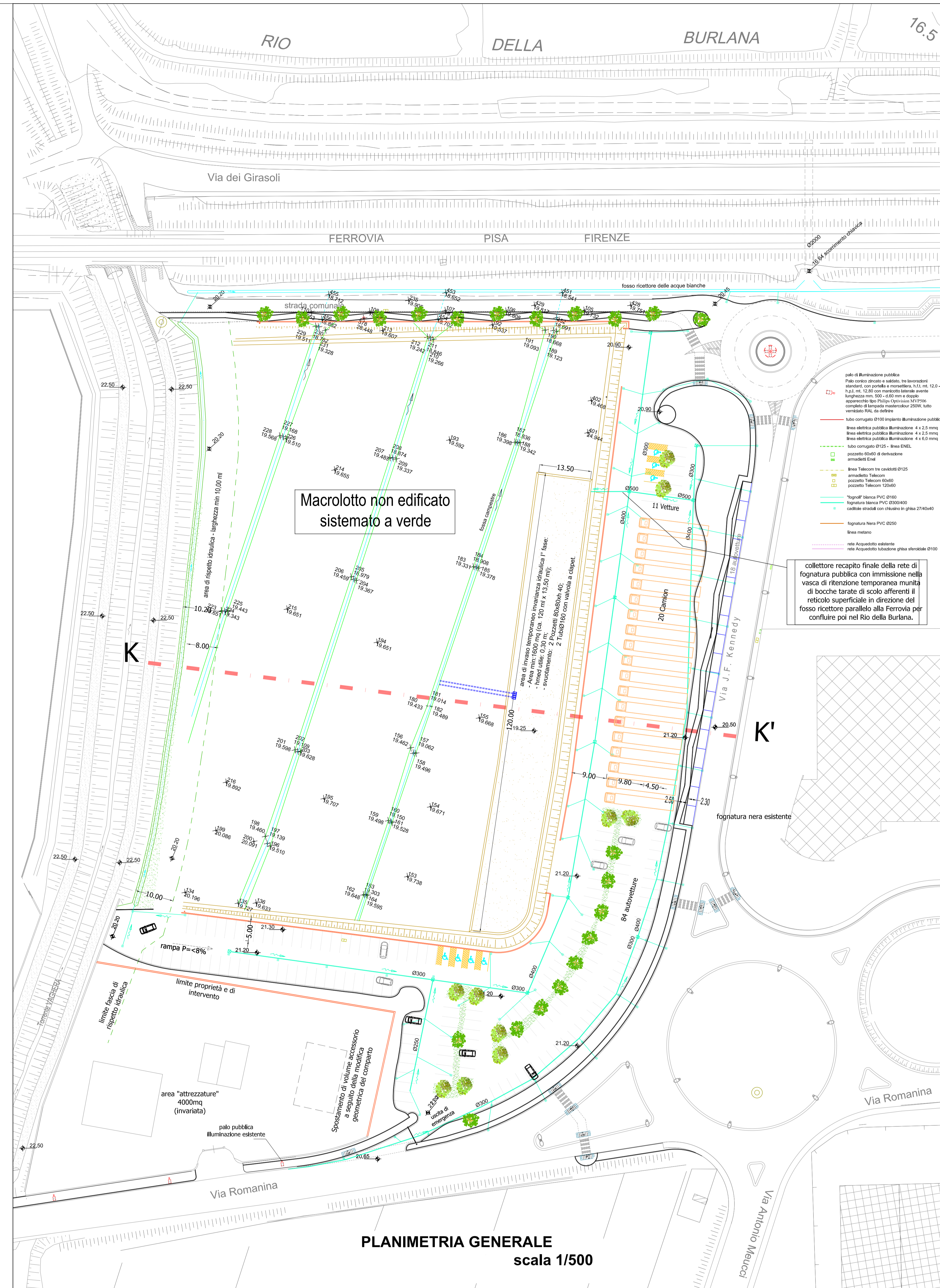
Verifica Invarianza Idraulica - I° Fase: Opere di urbanizzazione realizzate con macrolotto non edificato
